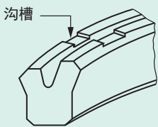
图13 非对称形防止背压沟槽型活塞密封圈
