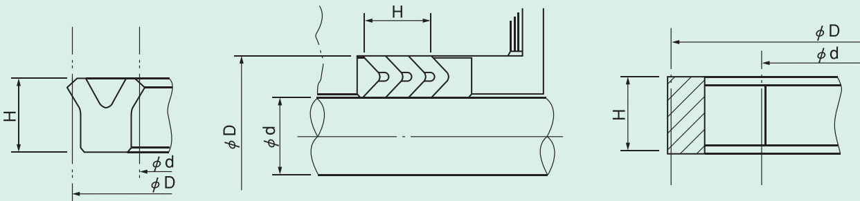
各种密封圈的高度（以公称高度即可）
