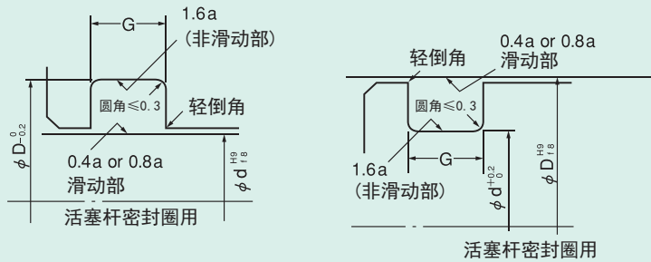
图2 U形密封圈腔尺寸
