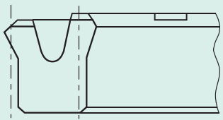
图12 非对称形防止背压沟槽型活塞密封圈（UHP、UNP、MLP系列）
