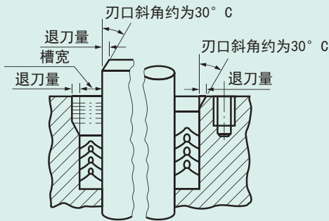
图4 V形密封圈插入部的倒角
