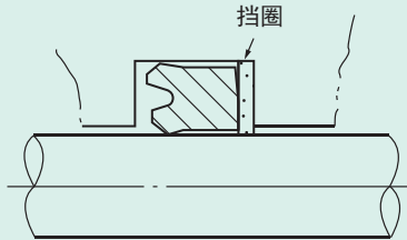
图7 同时使用挡圈
