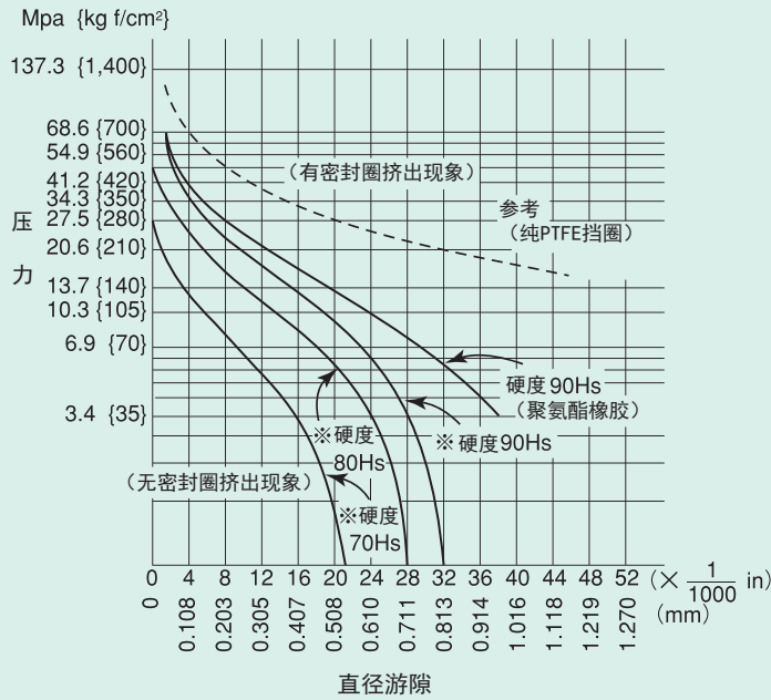
图8 密封圈挤出极限曲线
